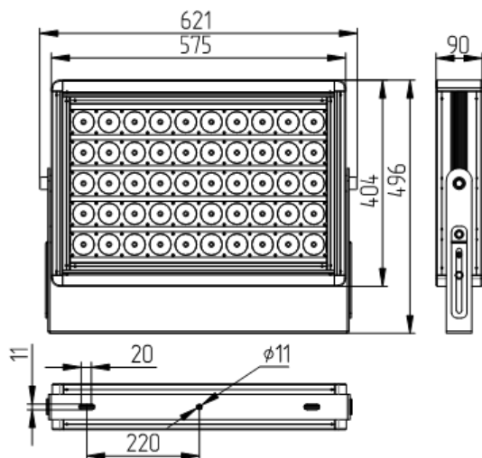
Рис.1 Габаритный чертеж прожектора Geniled Solar 500
