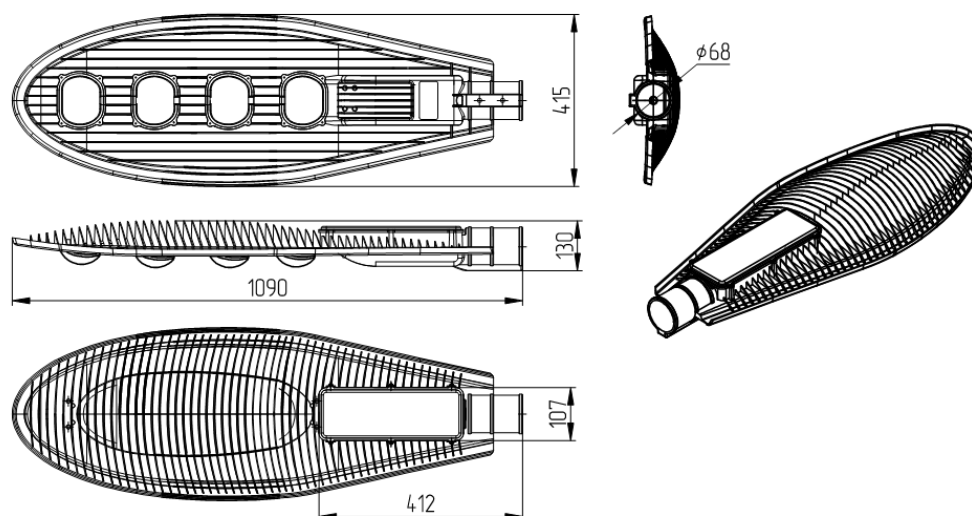
Рисунок 3 – Габаритный чертеж светильника Geniled Консоль 200W.
