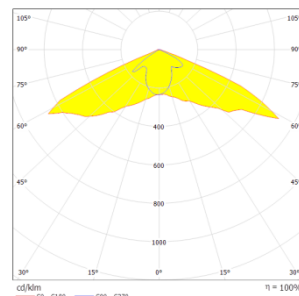
Рисунок 2 – Световое распределение светильника Geniled Консоль 200W.
