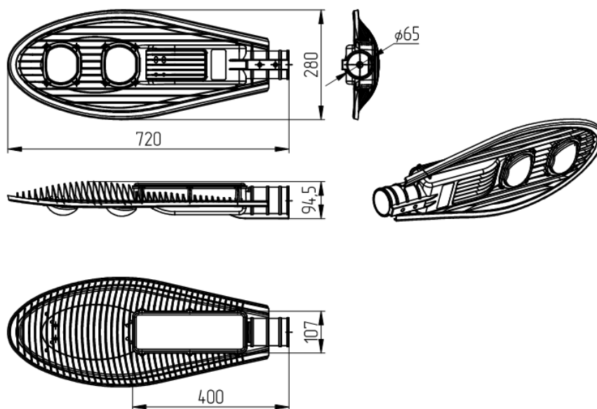
Рисунок 3 – Габаритный чертеж светильника Geniled Консоль 100W.
