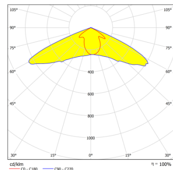
Рисунок 2 – Световое распределение светильника Geniled Консоль 100W.
