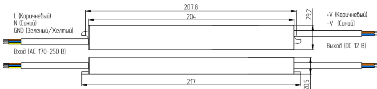
Рисунок 2 – Габаритный чертеж.
